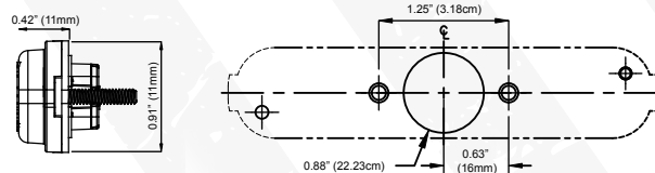
Stud Dimensions
